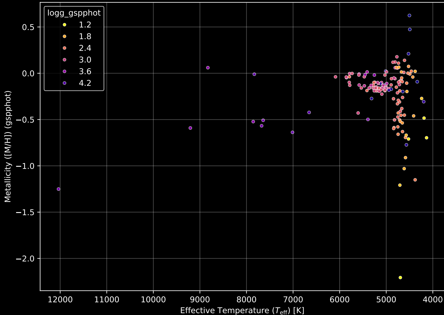
APOGEE DR17 Field: [225-12] Stellar Population Parameters (n= 152)
